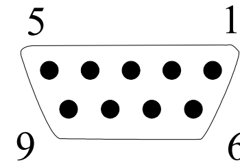
DB9-Hembra (Vista Frontal)
