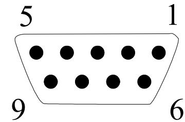
DB9-Hembra (Vista Frontal)
