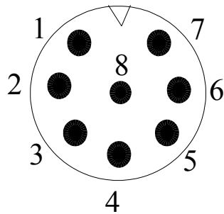
DIN 8 (Vista Trasera-soldadura)
