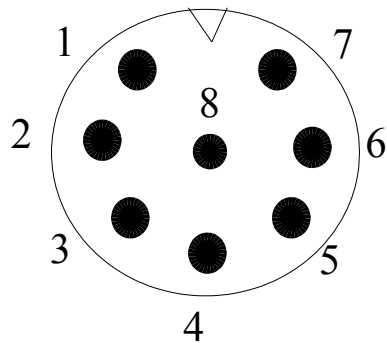
DIN 8 (Vista Trasera-soldadura)
